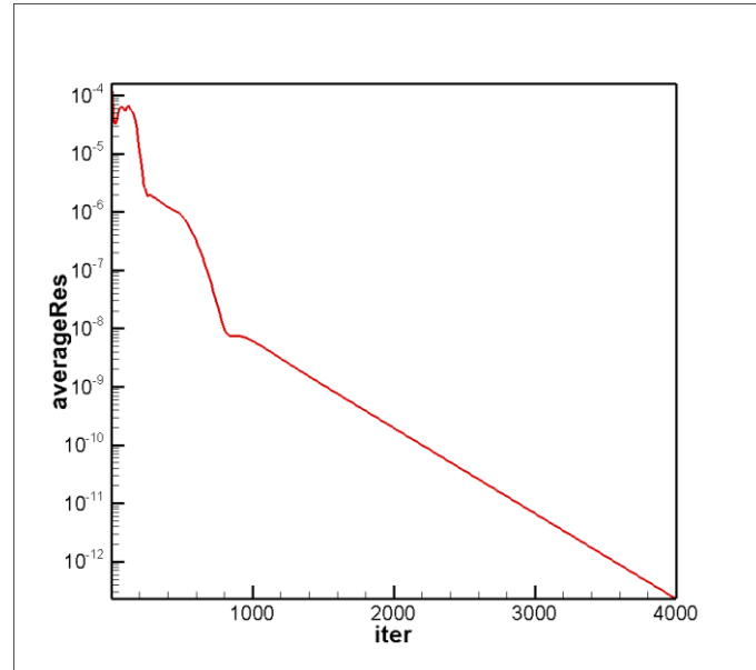
图 2 残差计算历程
