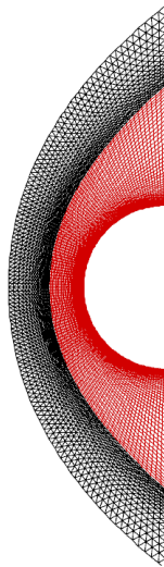
图 1 二维高速圆柱网格（红色为结构网格，黑色为非结构网格）
