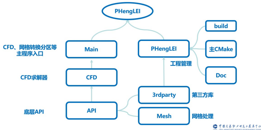
图 7 文件结构
