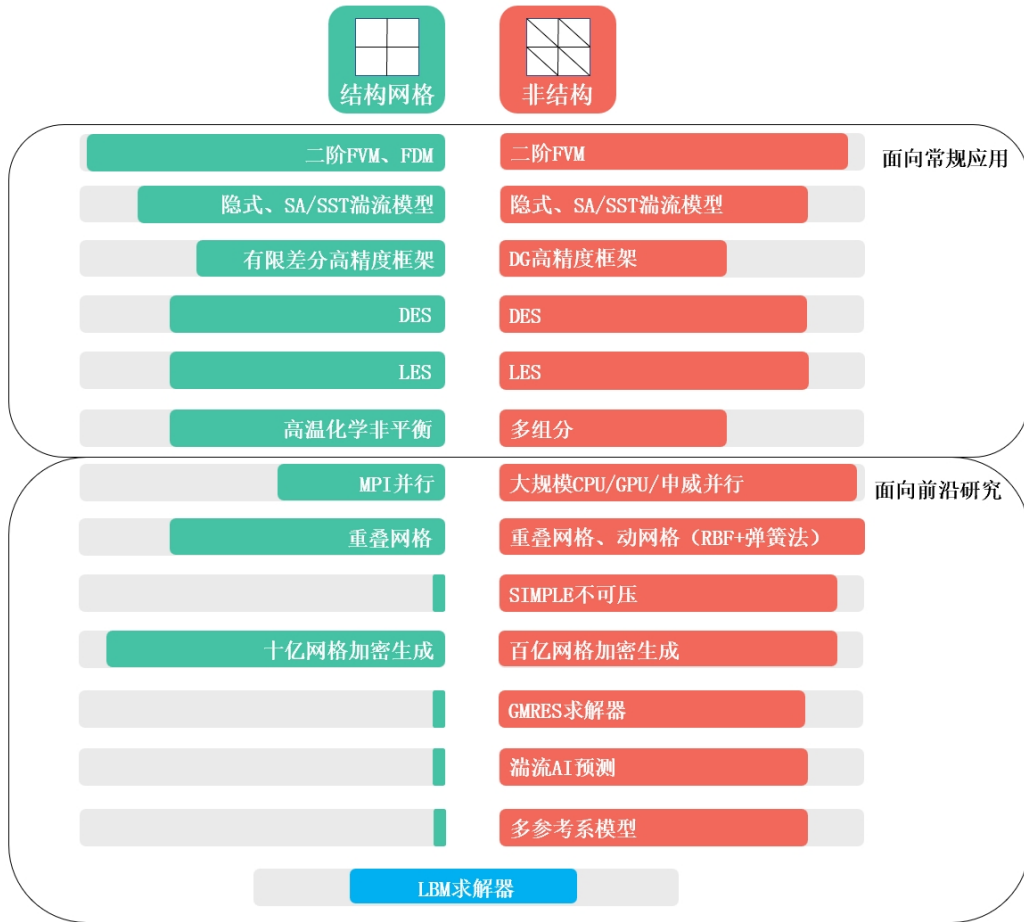
图 1 软件功能
