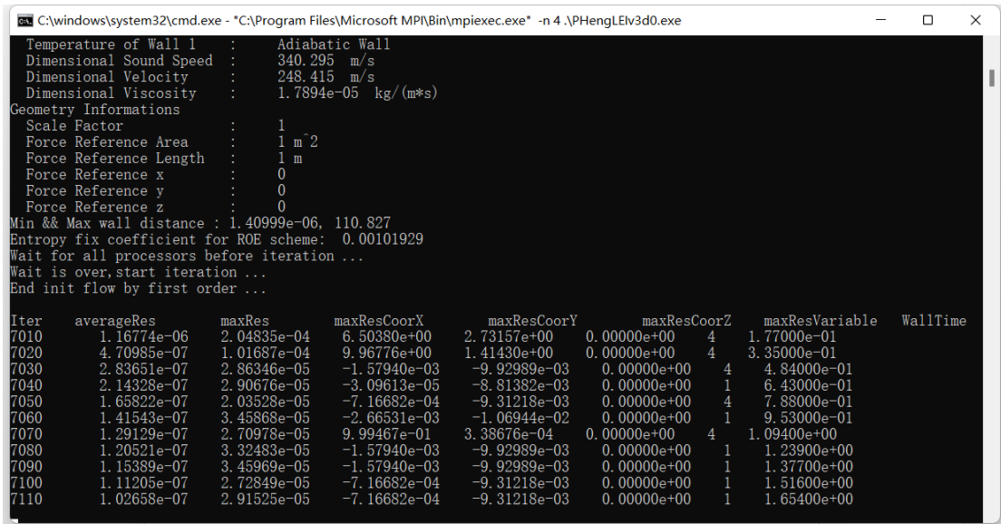
图 17 运行界面
